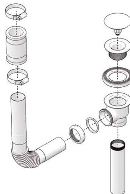
ENSEMBLE DRAIN & TROP-PLEIN EN LAITON
