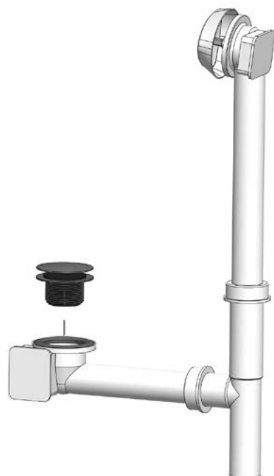
ENSEMBLE DE DRAIN & TROP-PLEIN PVC
