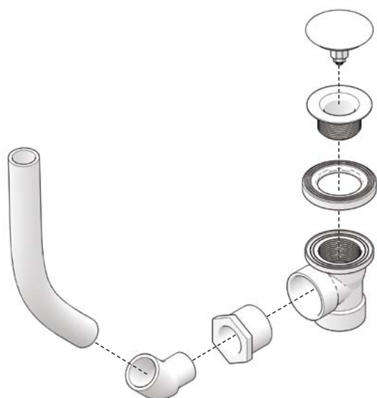
ENSEMBLE DE DRAIN & TROP-PLEIN PVC
